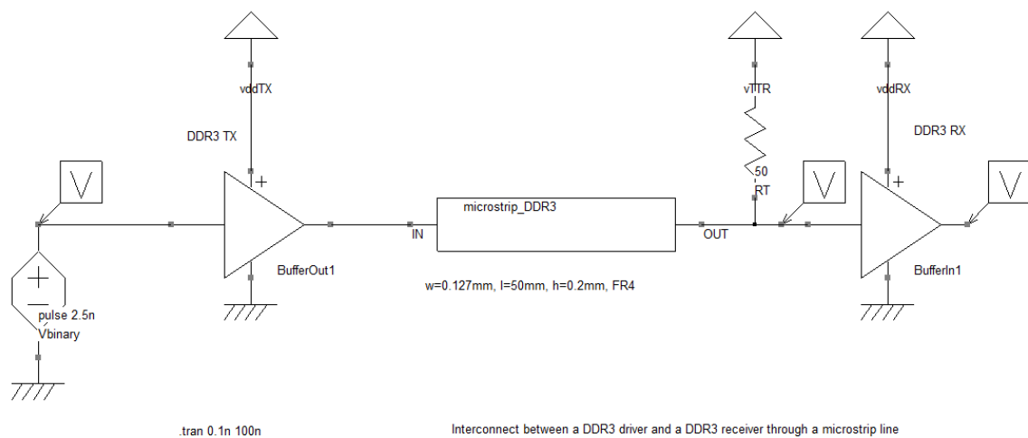
Figure 3- 44: Model of a DDR3 memory link (\examples\transient\DDR3_link_400MHz.sch)
